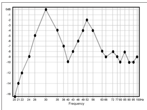
Figure 16. Deux pics de réponse
