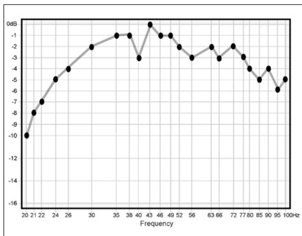
Figure 20. Réponse idéale, pas besoin d'égaliser
