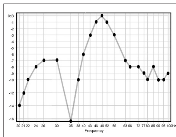
Figure 17. Chutes de réponse suivant ou précédant un pic
