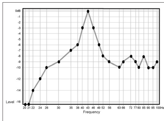
Figure 10. Exemple de résultat de test une fois tous les points reliés
