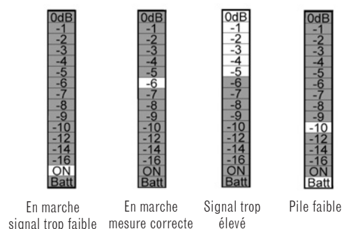
Figure 4. Indications de l'afficheur du sonomètre
