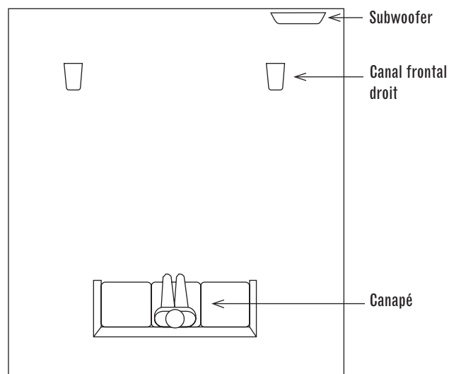
Figure 1. Dans cet exemple, le caisson de graves est placé derrière l'enceinte satellite de droite pour simuler la place habituellement dévolue aux basses dans un orchestre et/ou renforcer l'impact des bandes son cinématographiques.
