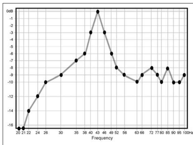
Figure 15. Un seul pic dominant
