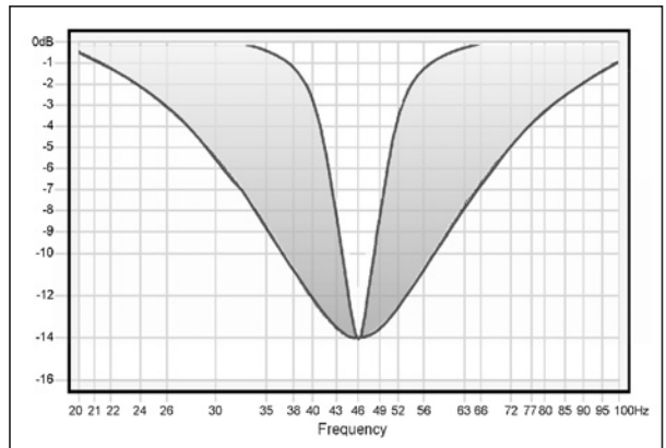
Figure 11. Influence de la largeur de bande
