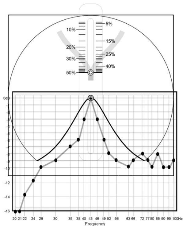
Figure 13. Positionnement du Sélecteur de largeur de bande
